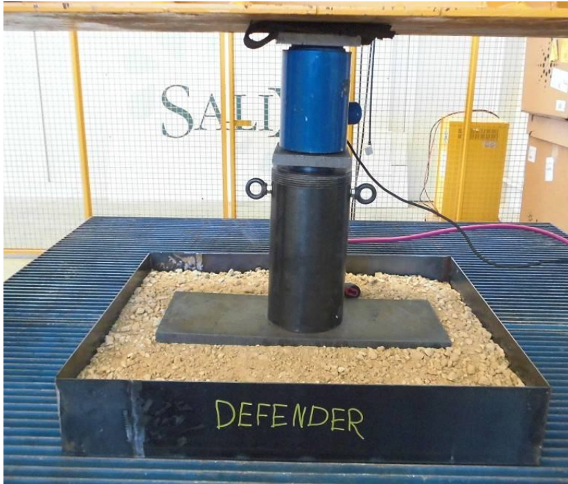
Resim 2: 0/12 kırma taş ile doldurulmuş 'DEFENDER' (sınırlanmış) numunesi yükleme testi detayı
