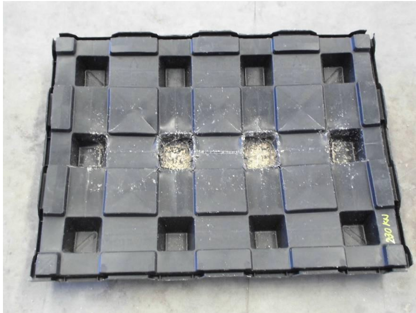
Resim 4: 0/12 kırma taş ile doldurulmuş 'DEFENDER' (sınırlanmış) numunesinin test sonunda kırılmış olan detayı (230 KN)
