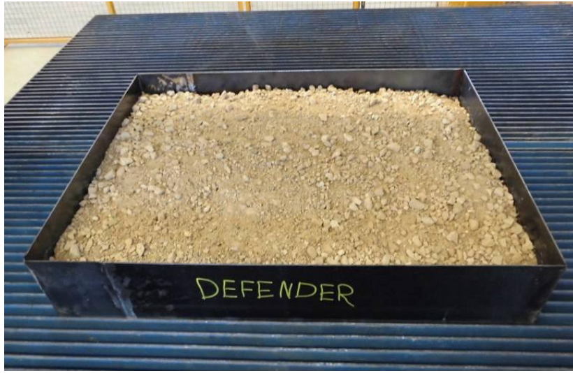
Resim 1: "DEFENDER" numunesi (sınırlanmış) 0/12 kırma taş ile doldurulmuş
