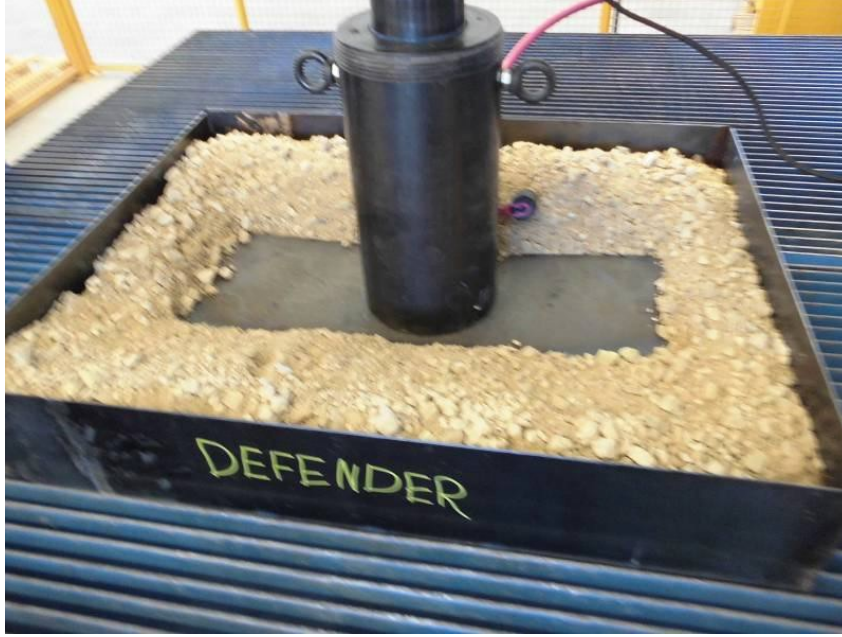
Resim 3: 0/12 kırma taş ile doldurulmuş 'DEFENDER' (sınırlanmış) numunesi yüklemeye detayı
