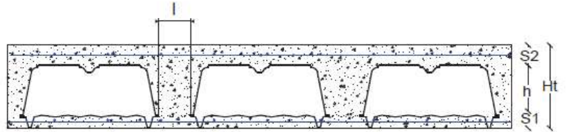
Kesit, TEK h: 20 cm, S1 ve S2: 10 cm, l: 20 cm
