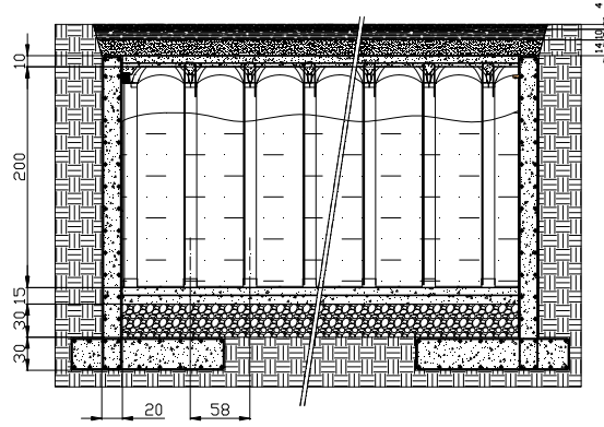
Şek.1 Enine kesit
