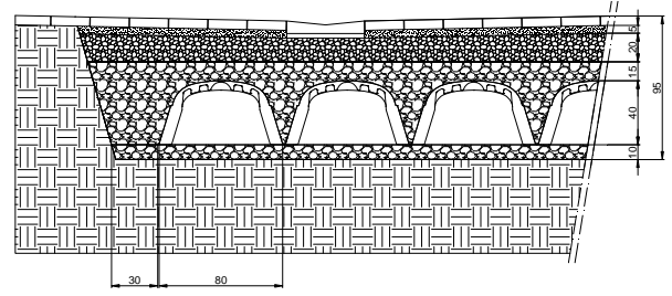
Şek.1 – Sistemin enine kesiti
