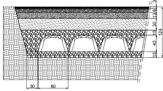
Şek.1 – Sistemin enine kesiti
